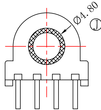
A-A SECTION
